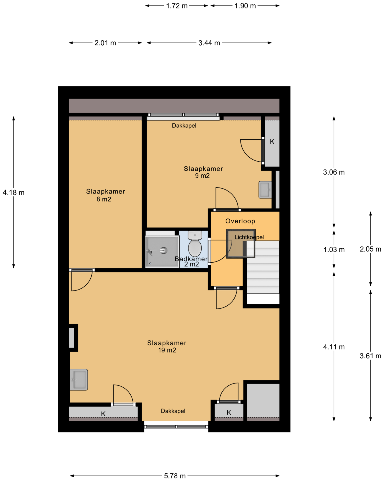
2e Verdieping
