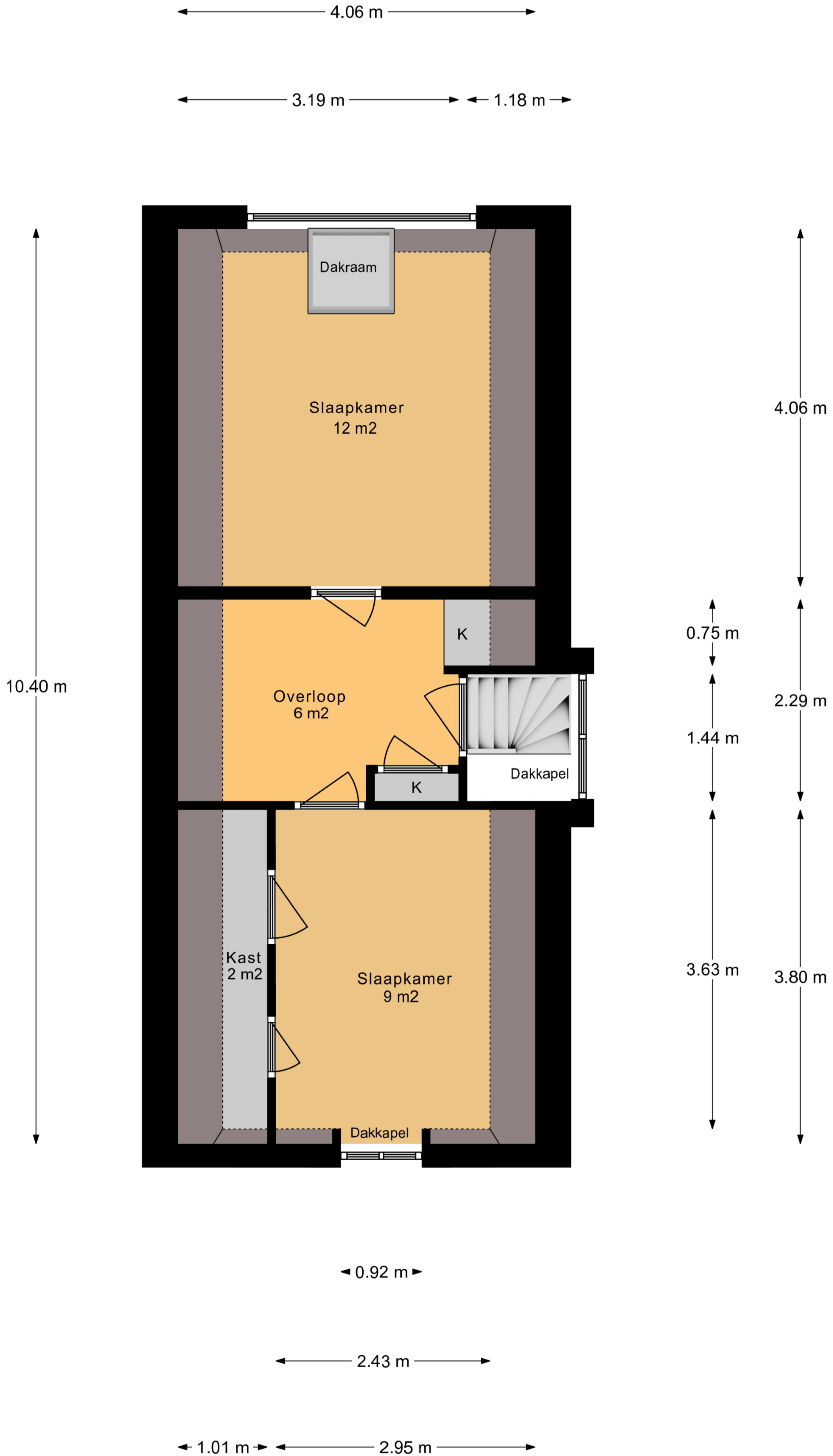
2e Verdieping
