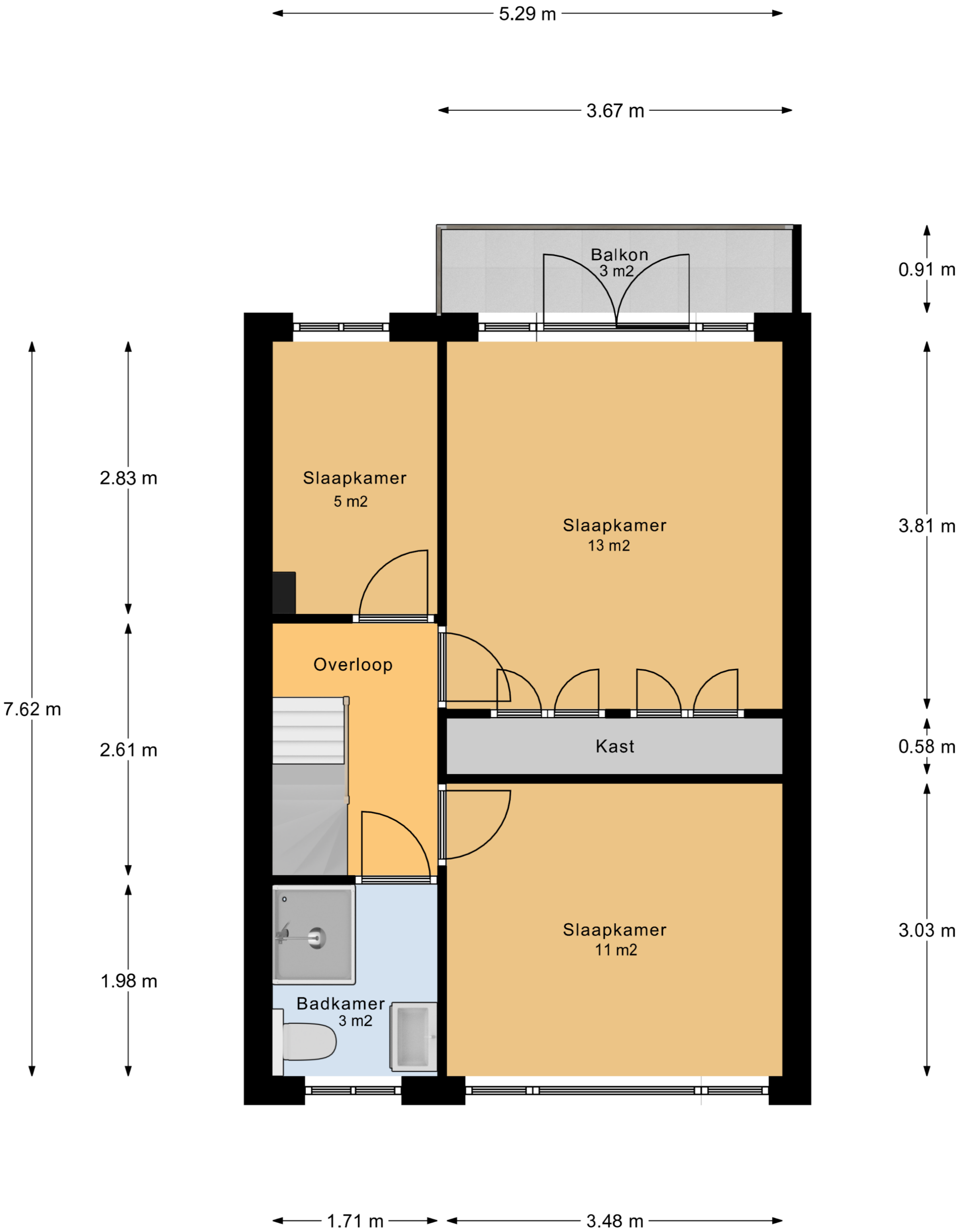
1e Verdieping
