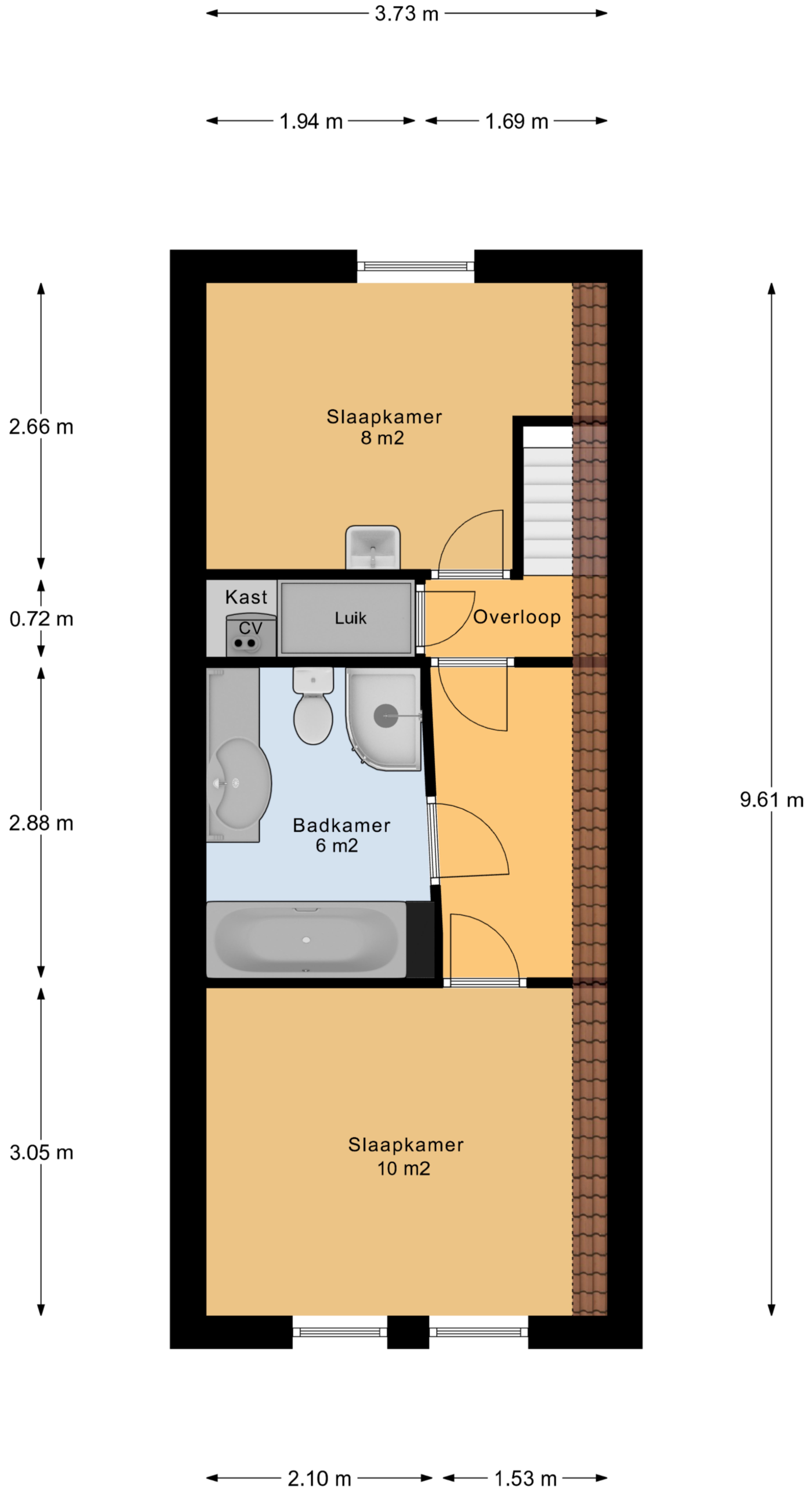
1e Verdieping
