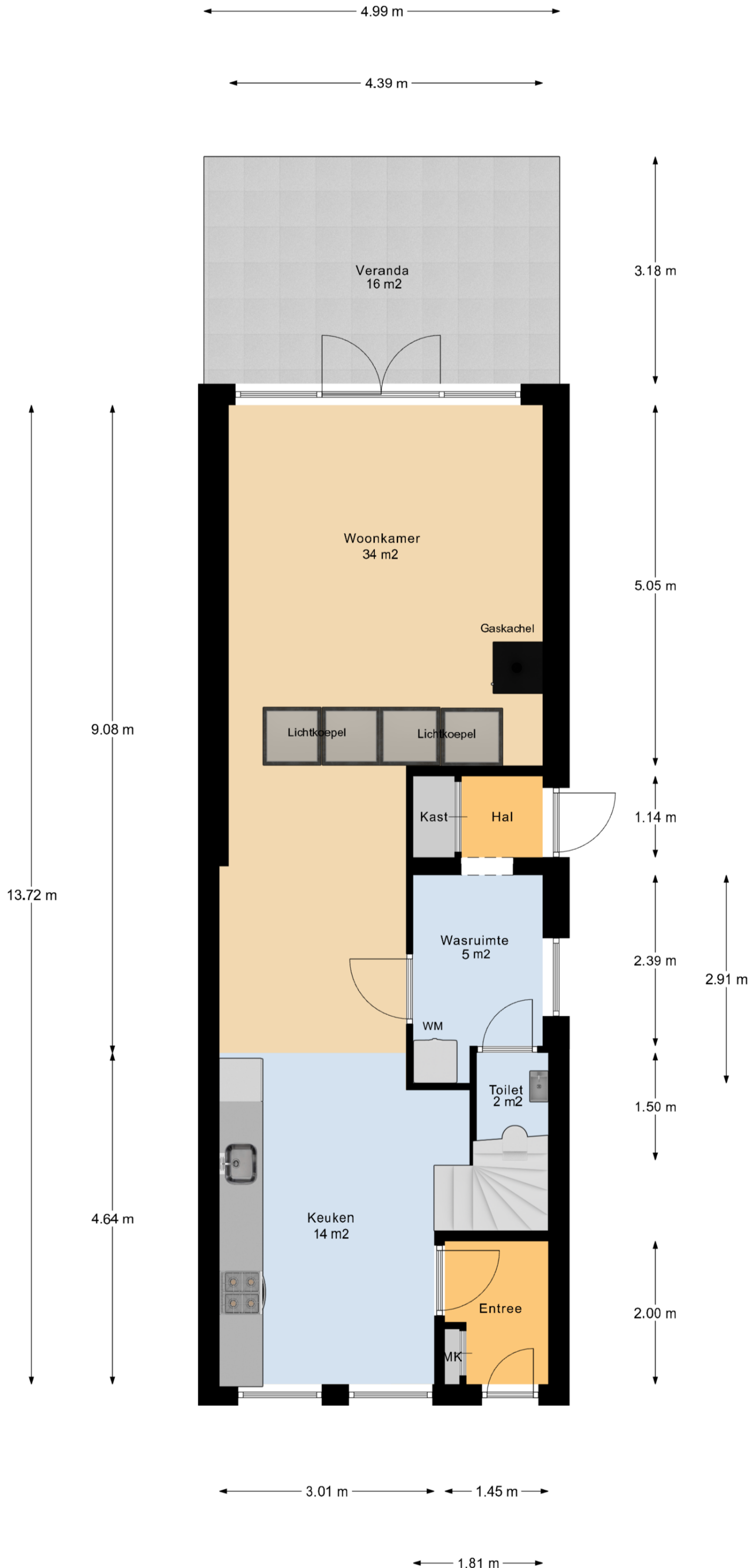
Begane Grond
