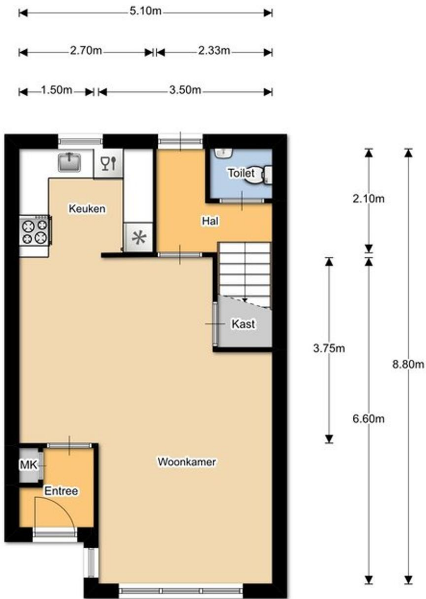
Begane grond
