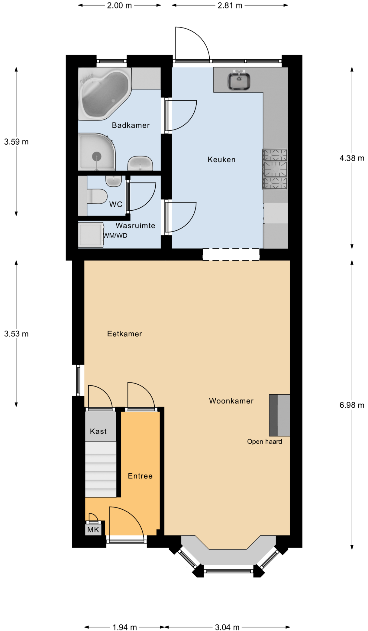
Begane Grond
