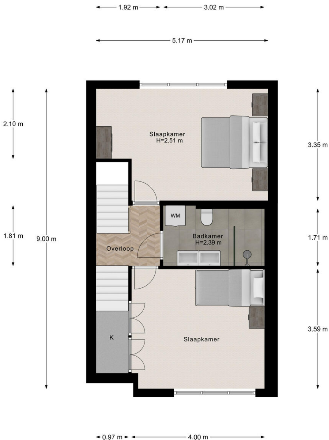
1e Verdieping
