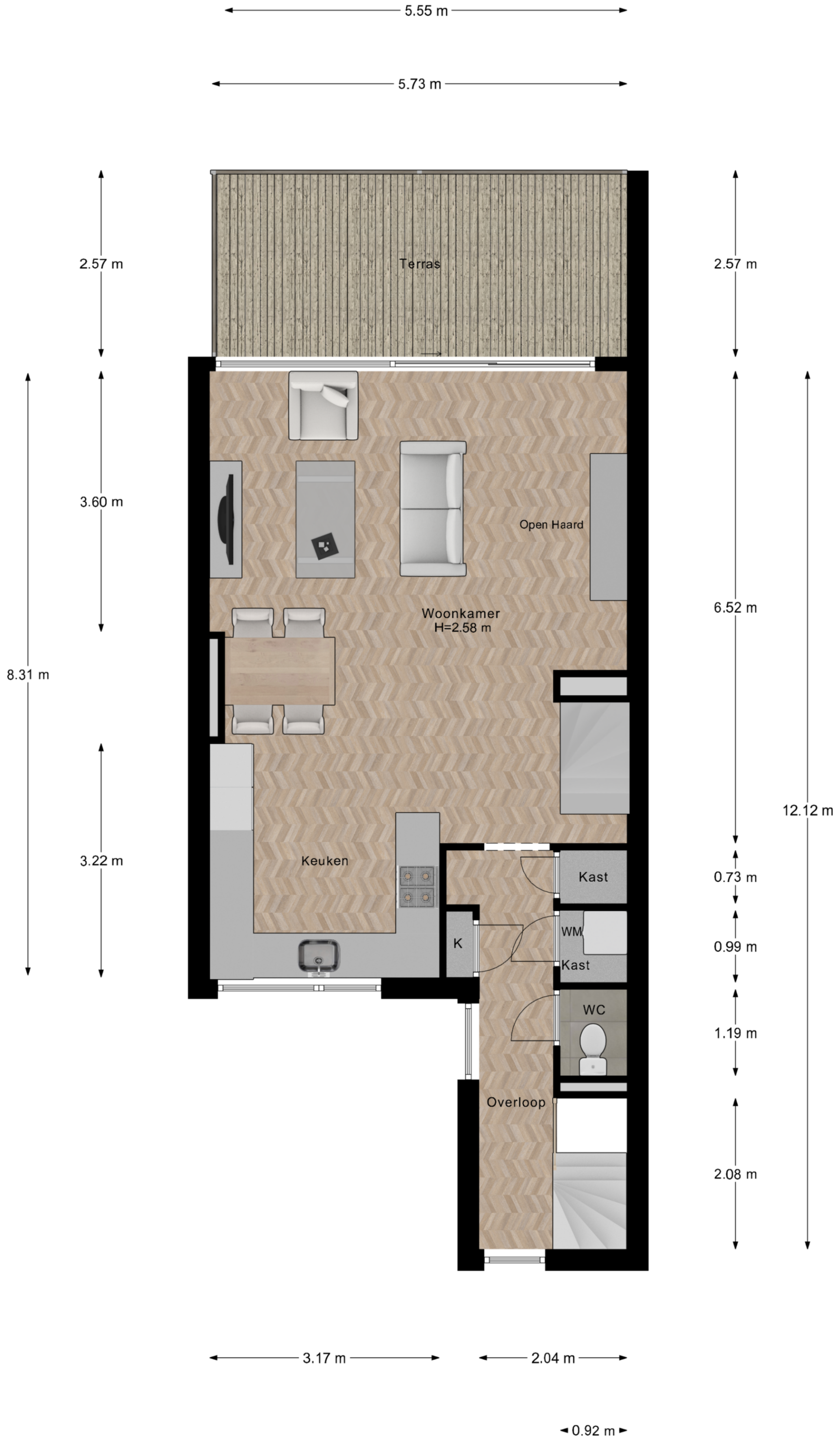
1e Verdieping
