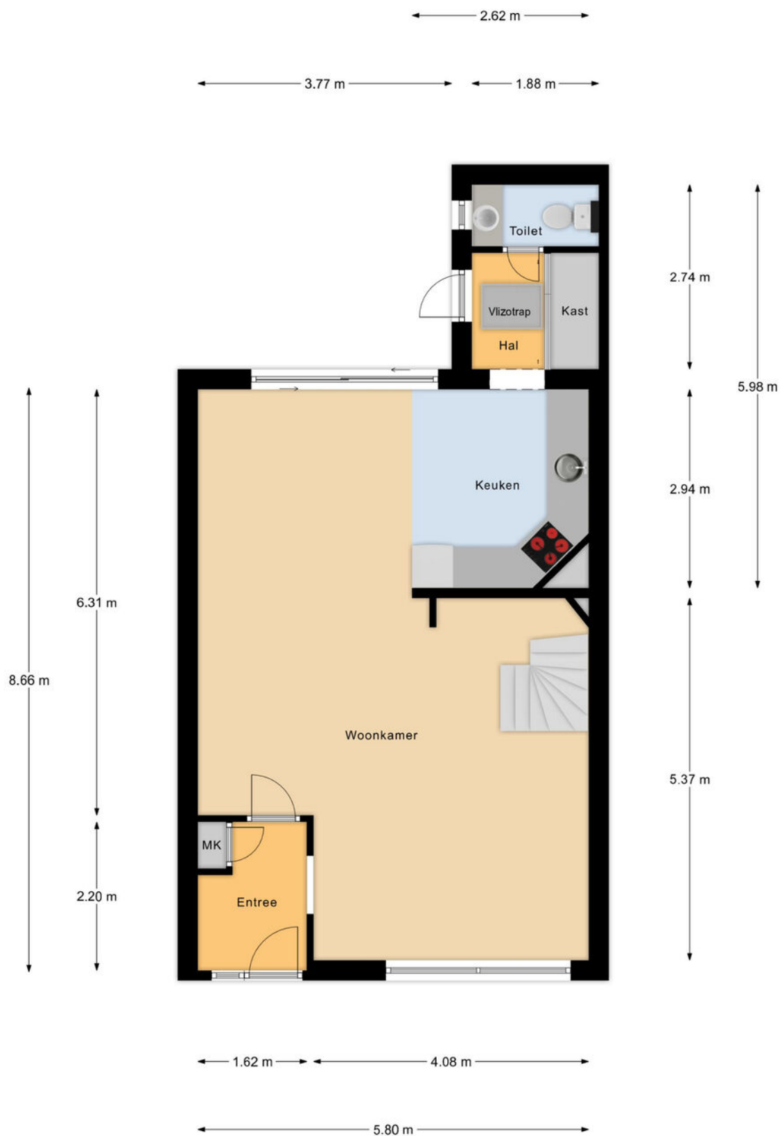
Begane Grond
