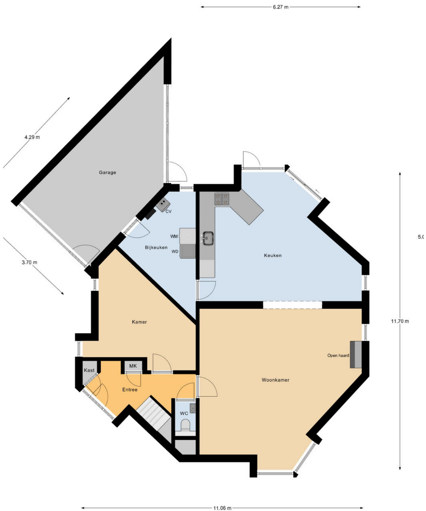
Begane Grond
