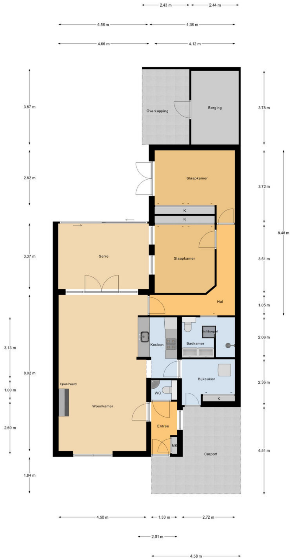
Begane Grond
