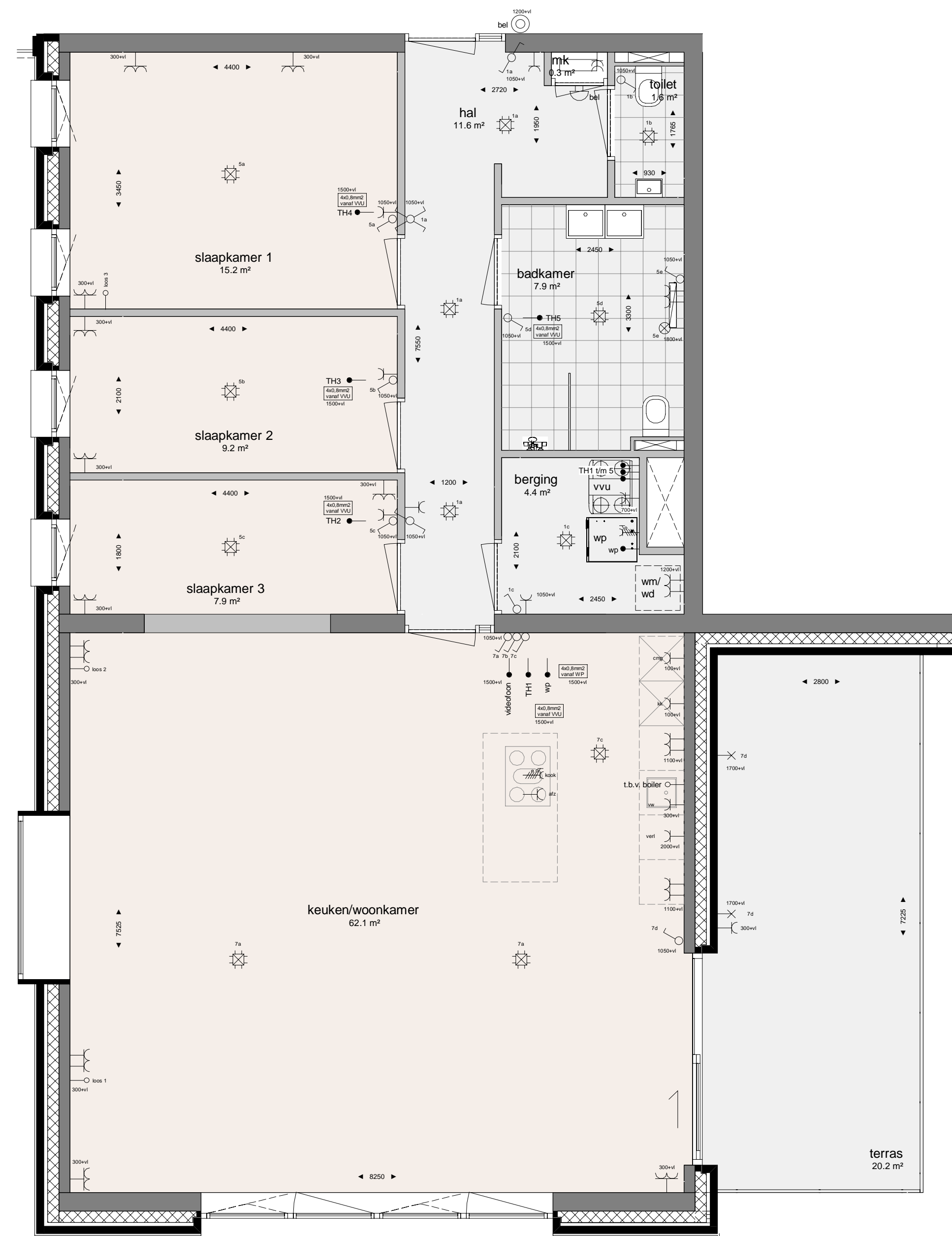
Appartement 3 - Laag 1 Schaal: 1:50
