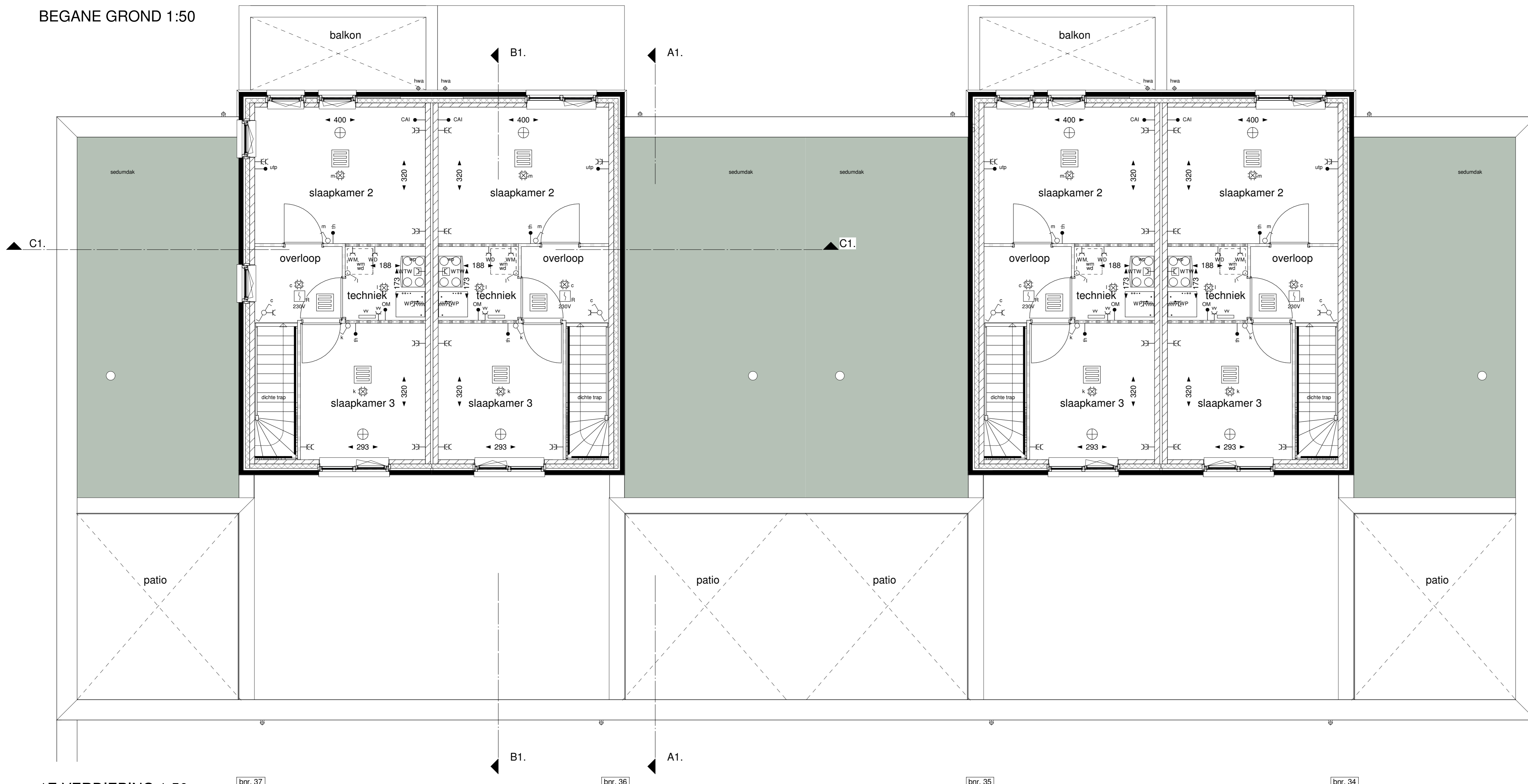
1E VERDIEPING 1:50
