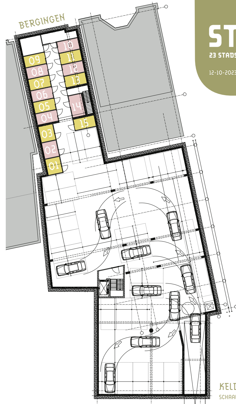
VERDIEPING 2 SCHAAL 1:200
