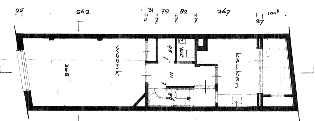
1e VERDIEPING
