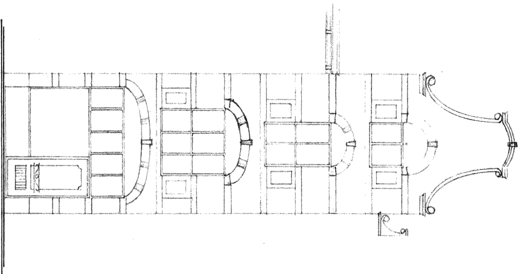
VOORGEVEL
