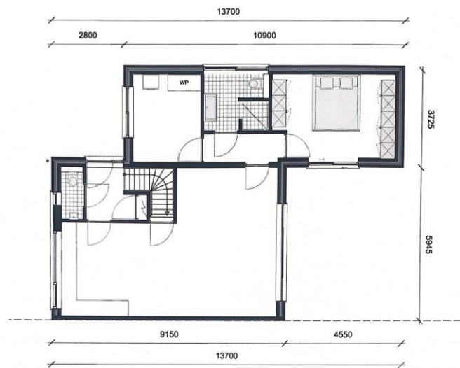
BEGANE GROND
