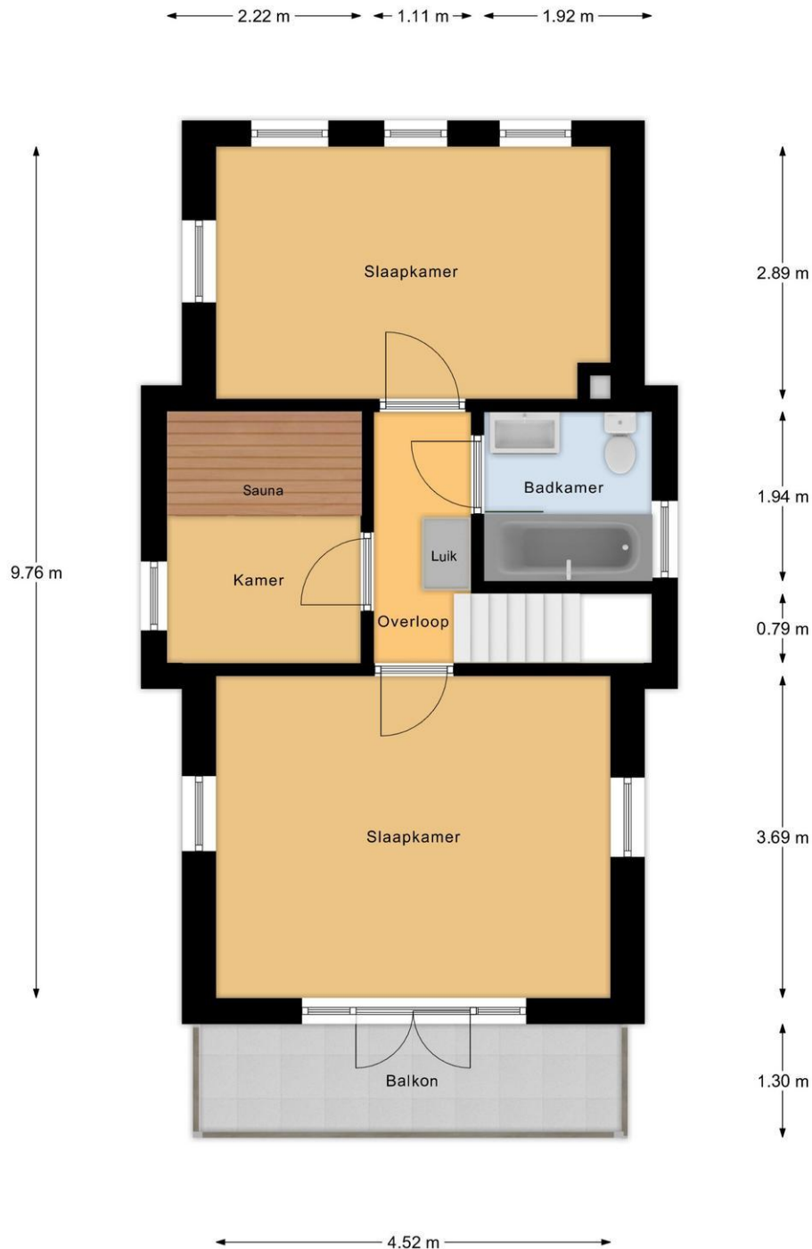
1e Verdieping
