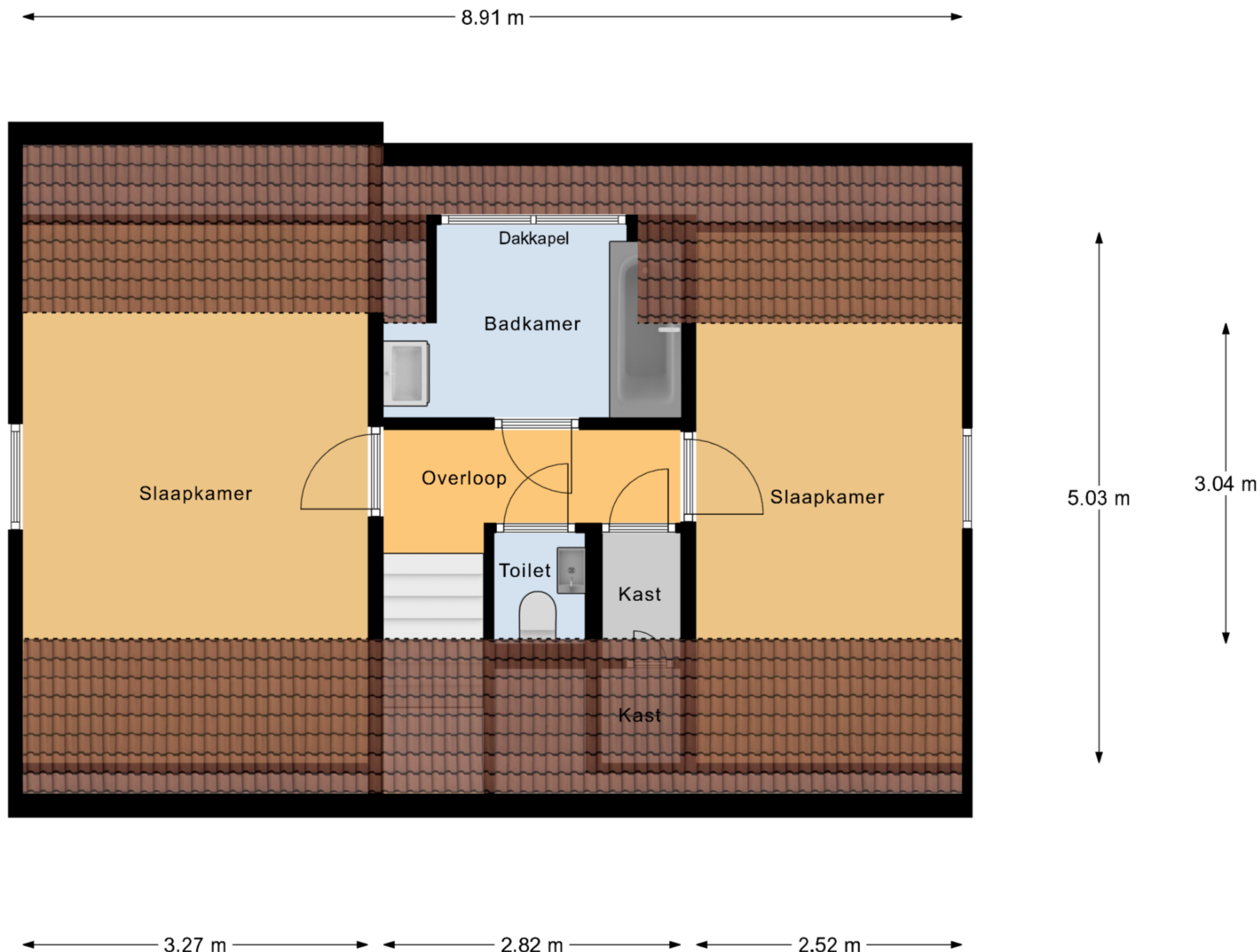
1e Verdieping
