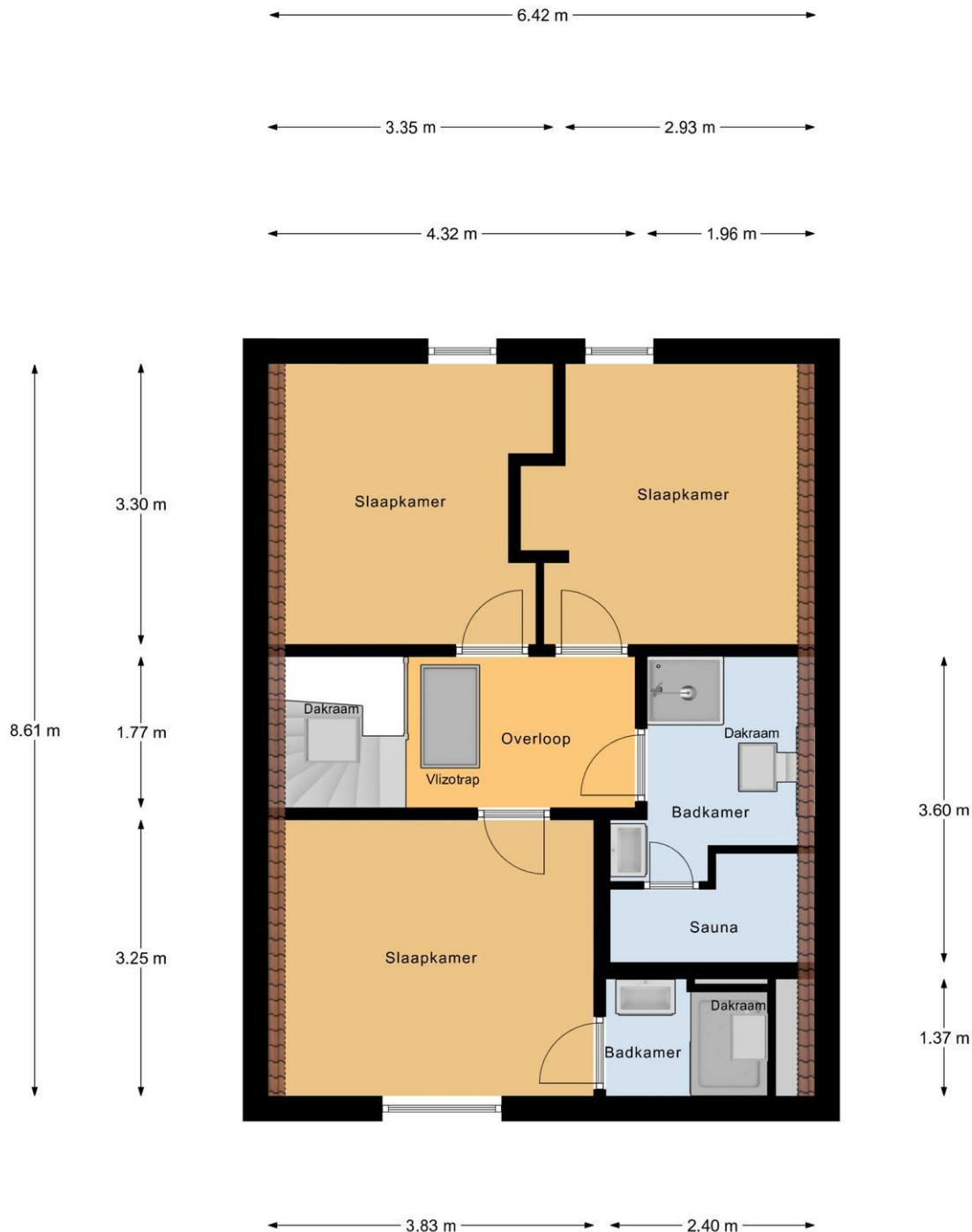
1e Verdieping
