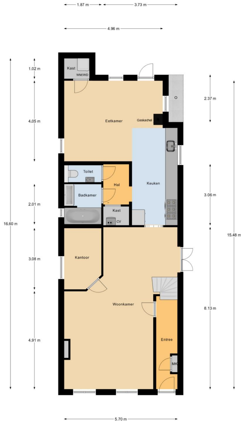
Begane Grond
