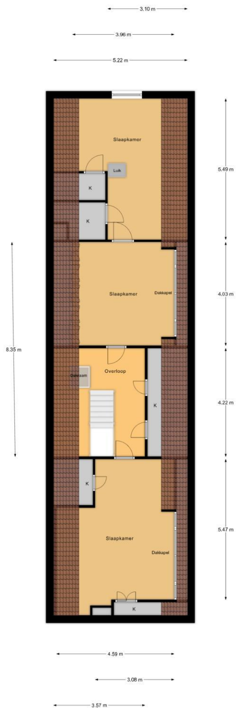
1e Verdieping
