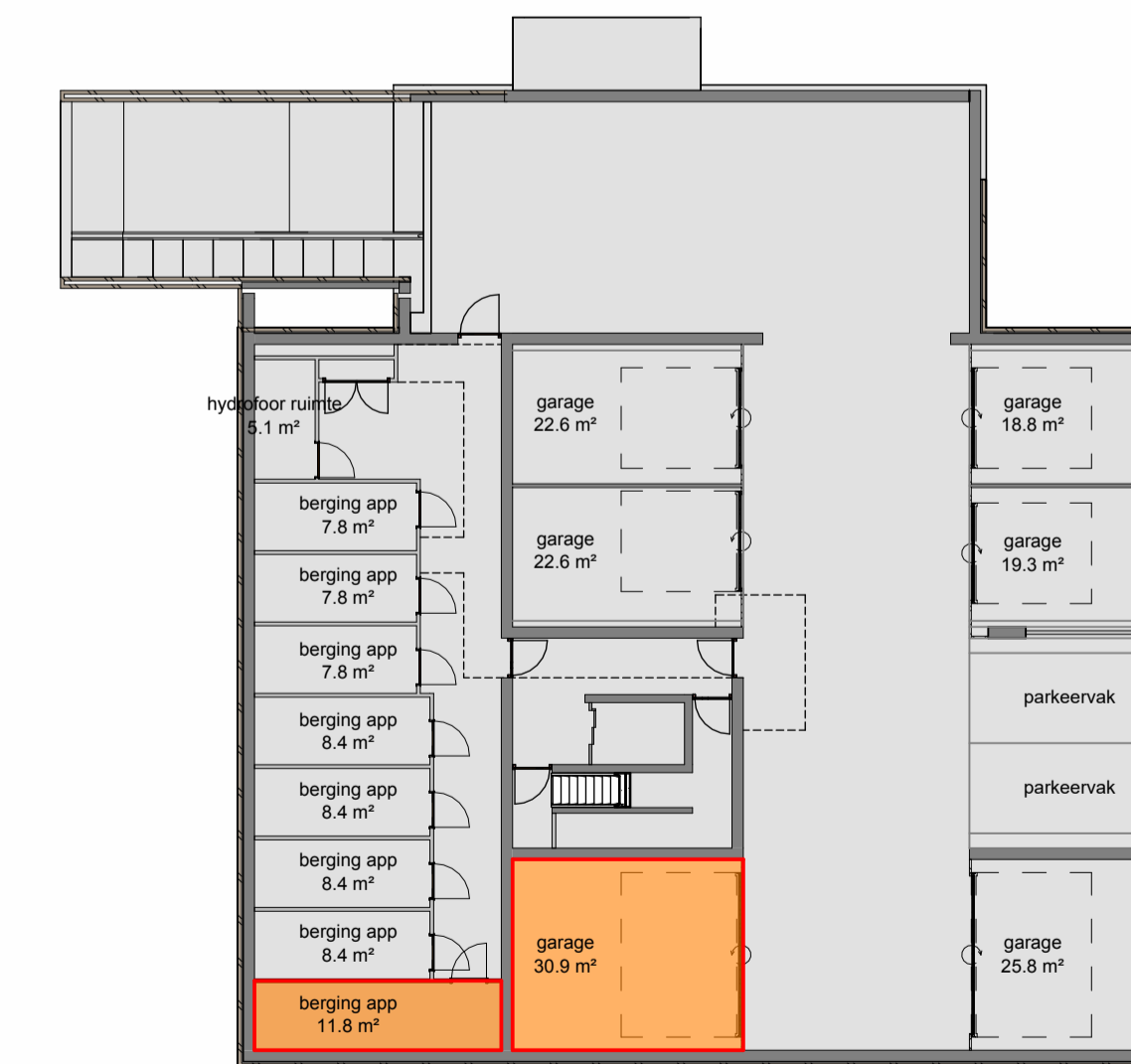
Overzichtsplattegrond kelder
