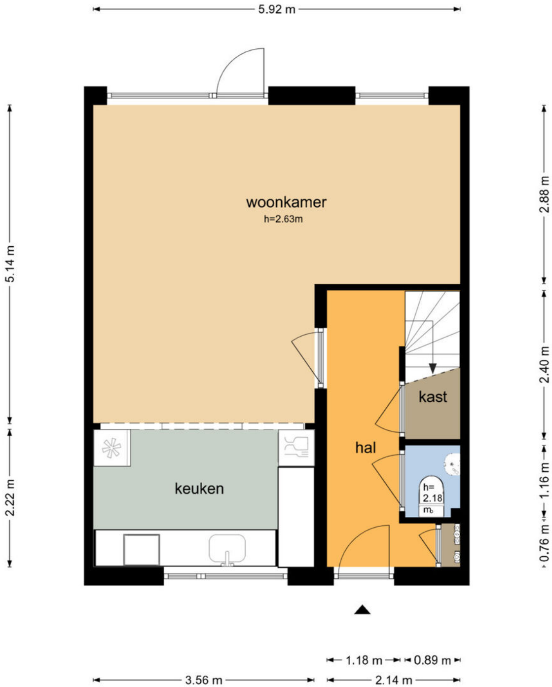
Westerzicht 183 - Vlissingen Begane Grond
