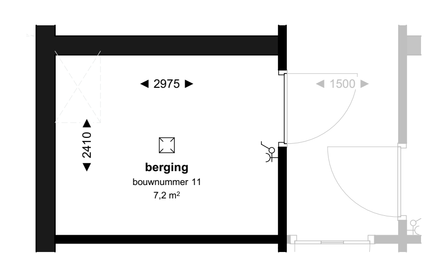
BERGING (kelder) 1:50
