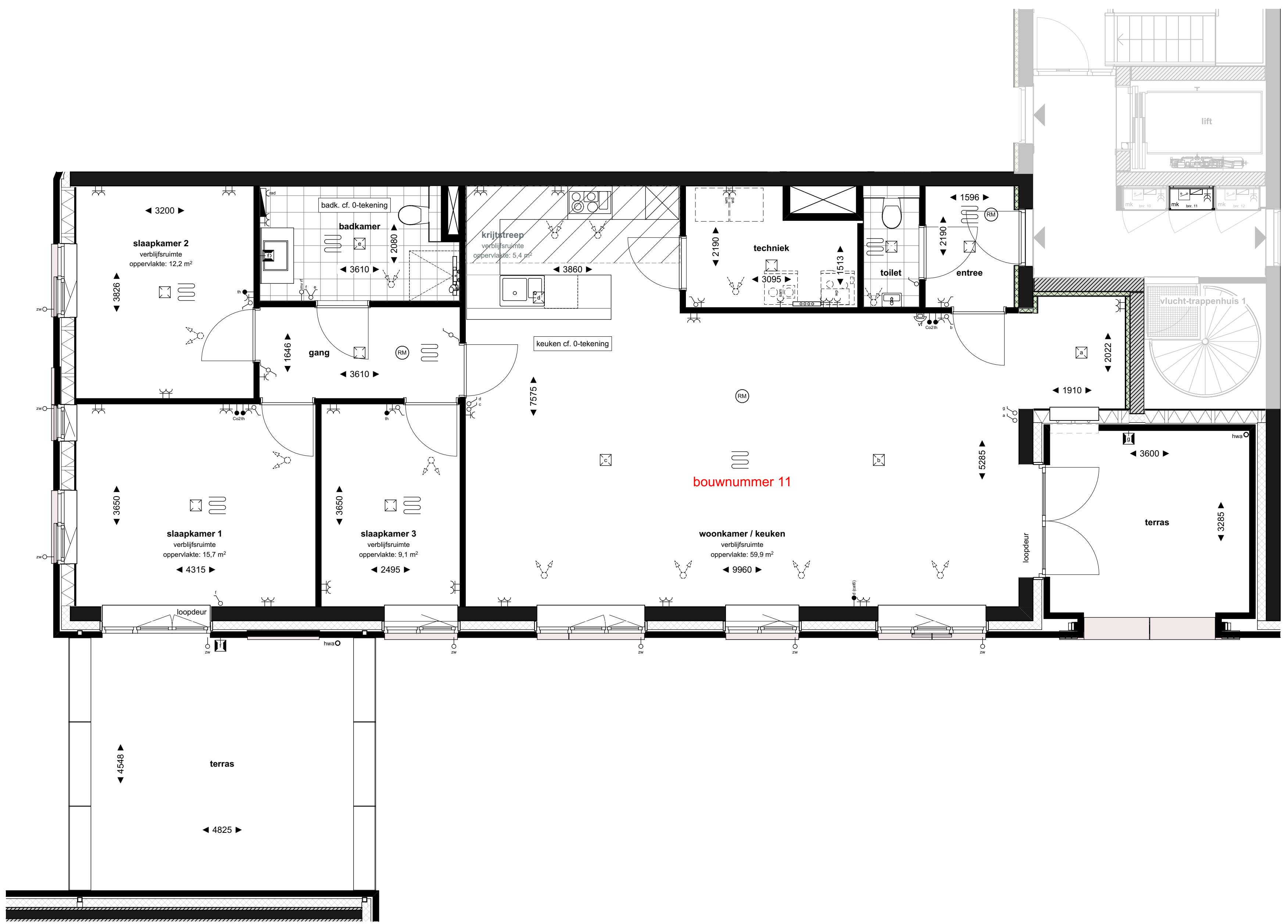
1e VERDIEPING 1:50
