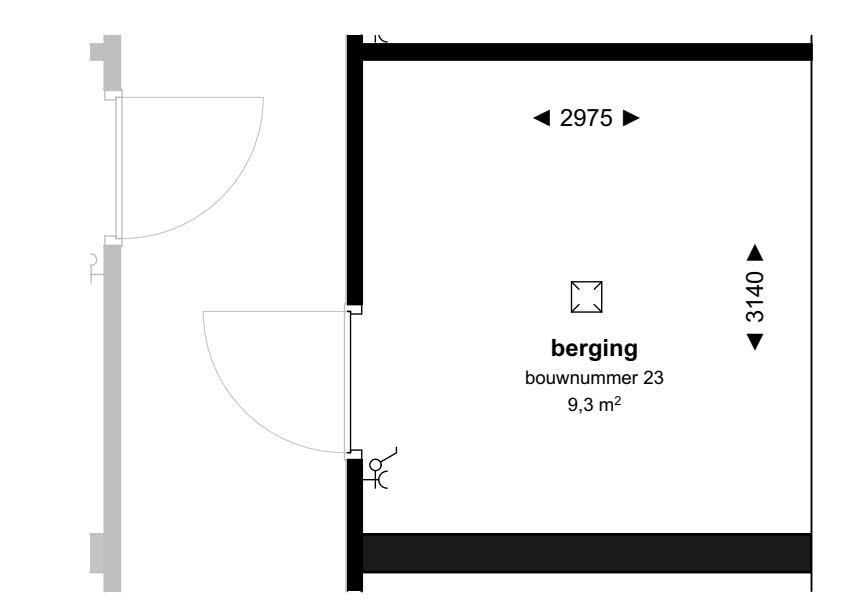
BERGING (kelder) 1:50
