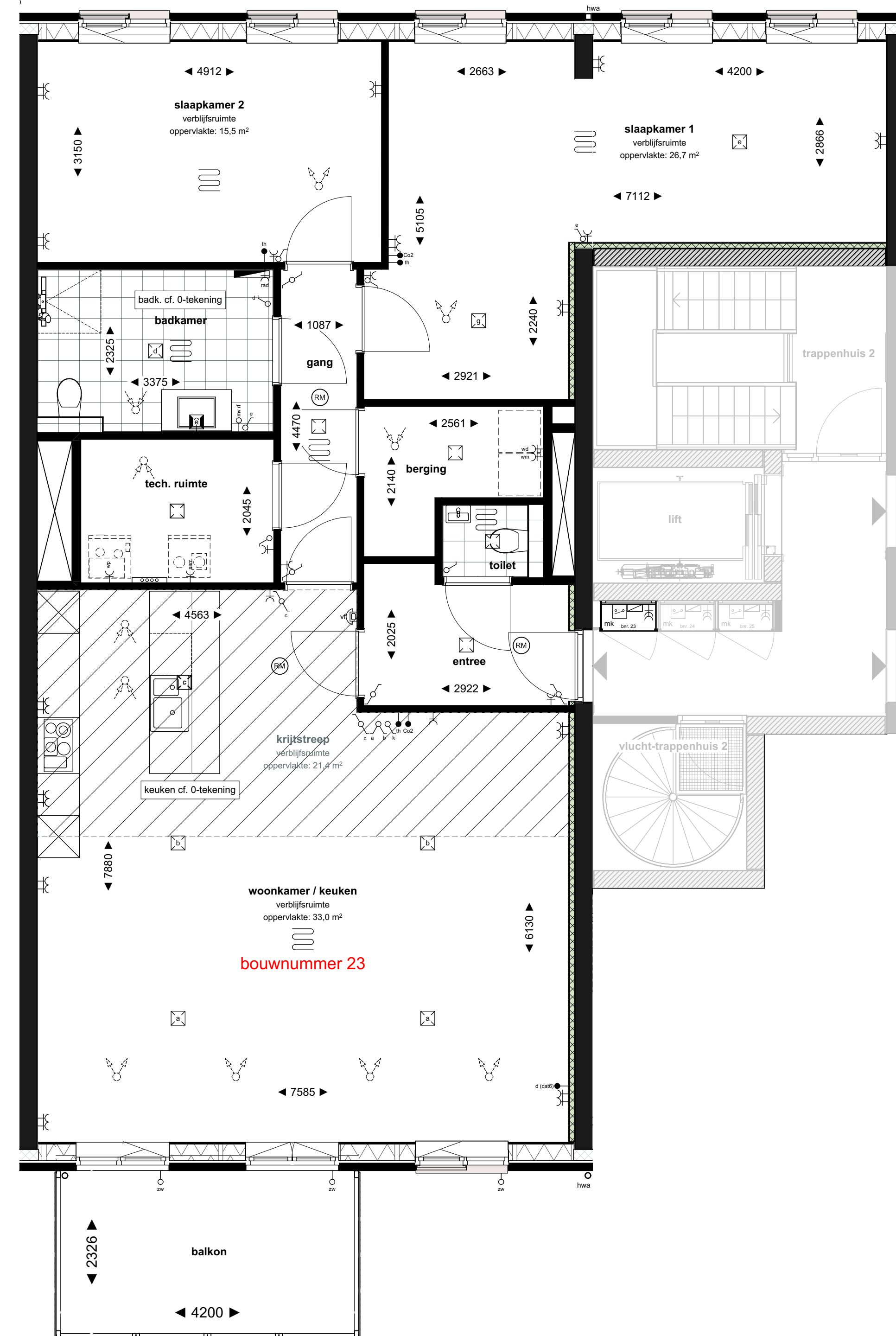
2e VERDIEPING 1:50
