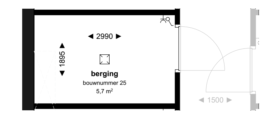
BERGING (kelder) 1:50
