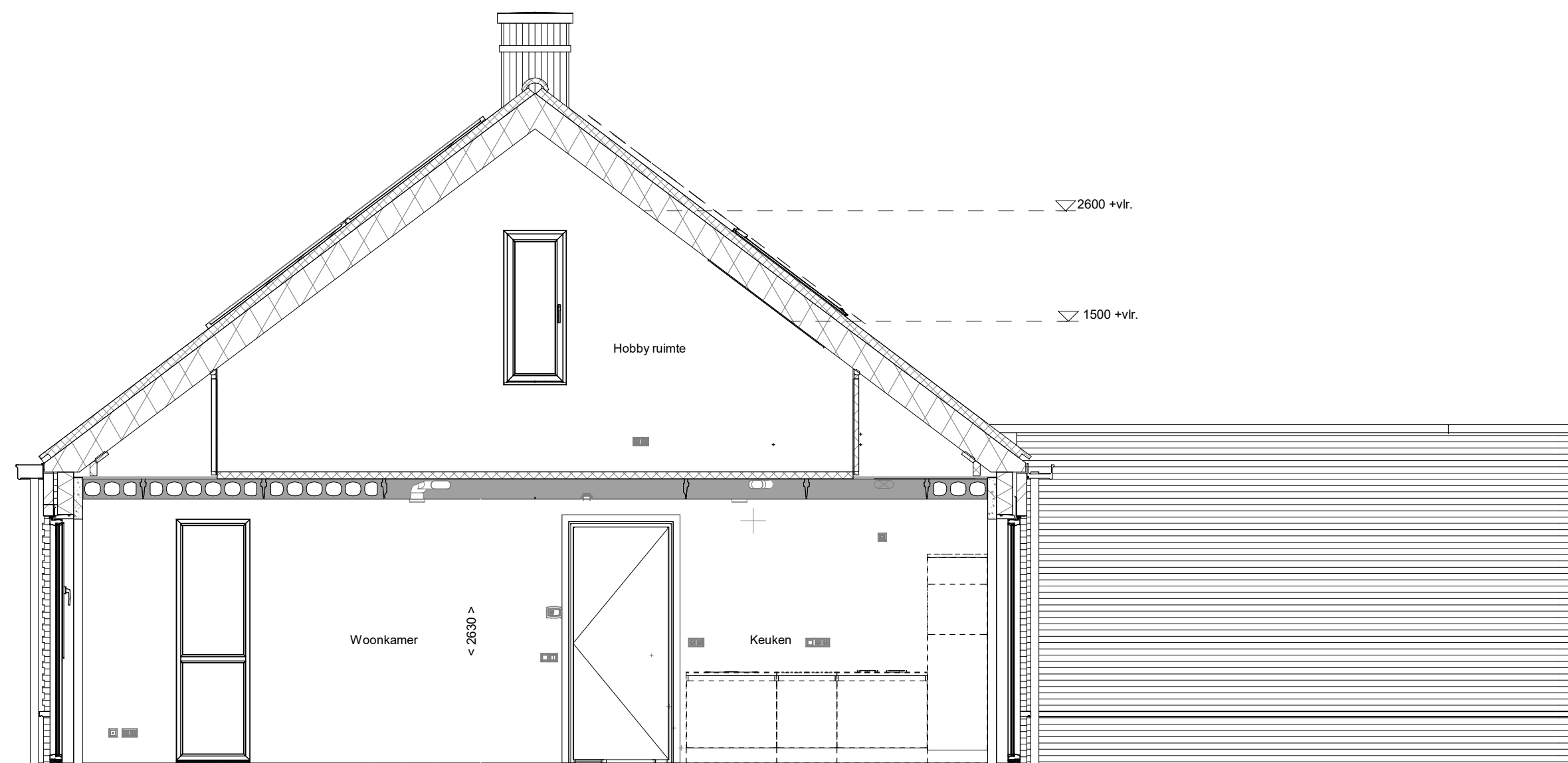
doorsnede A-A 1 : 50
