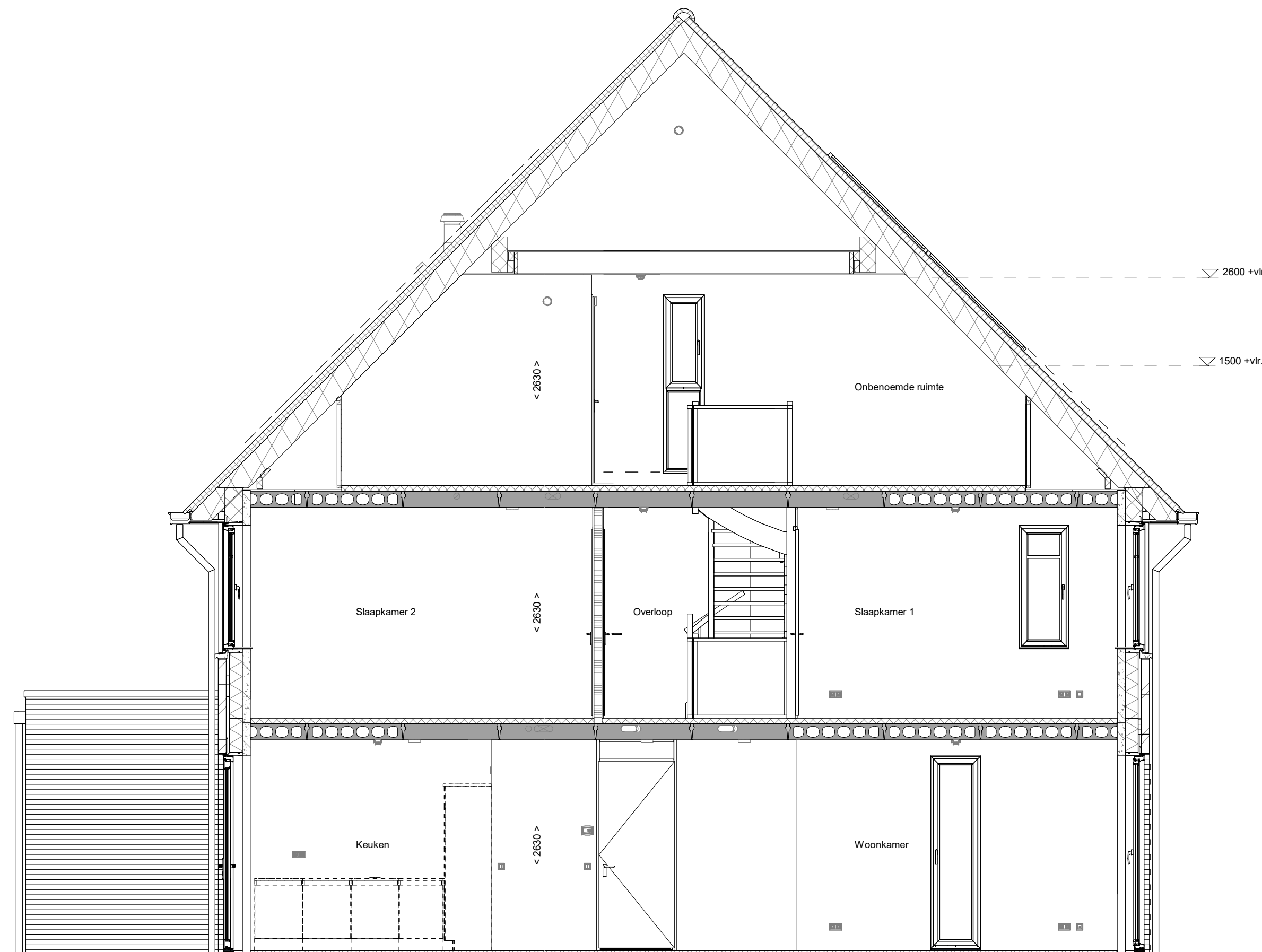
doorsnede A-A 1 : 50
