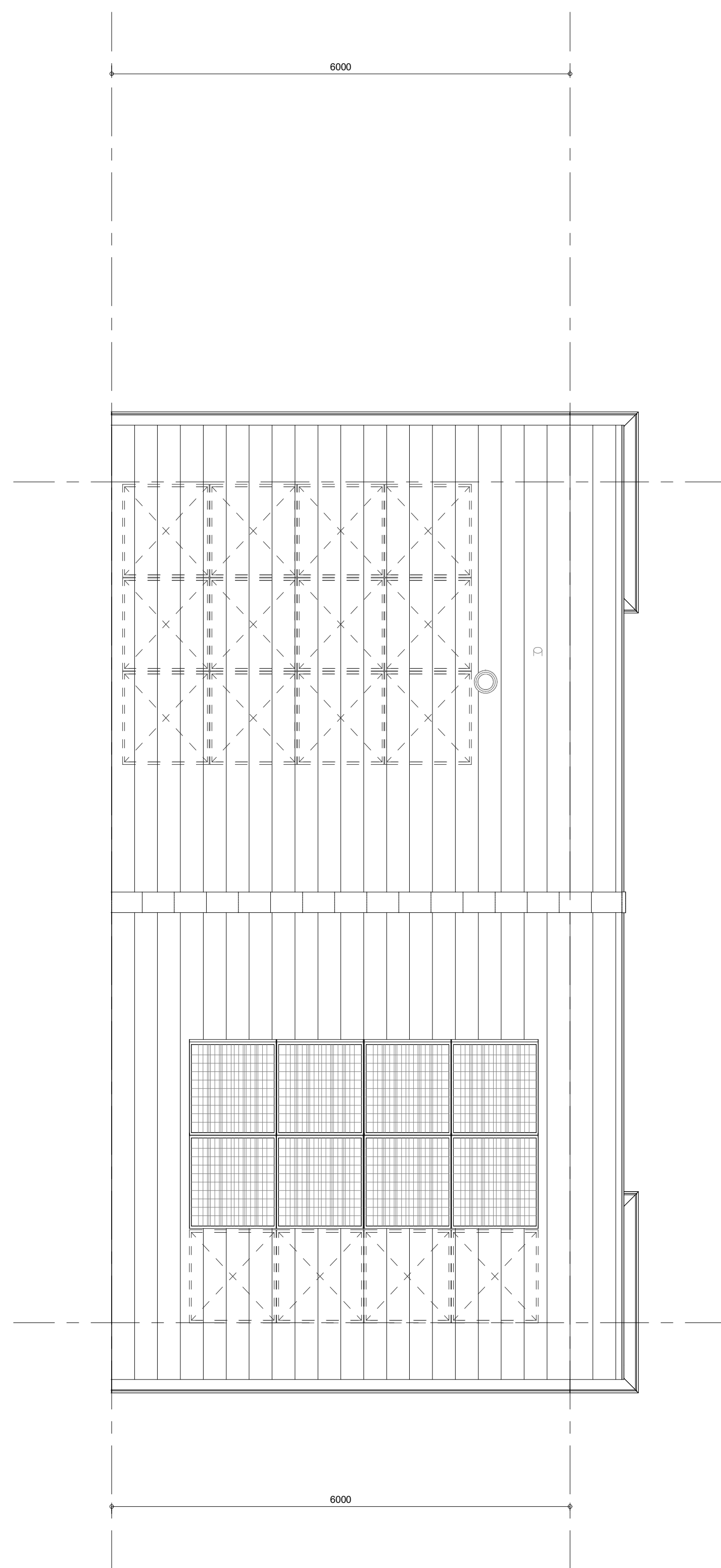
Dakaanzicht 1 : 50
