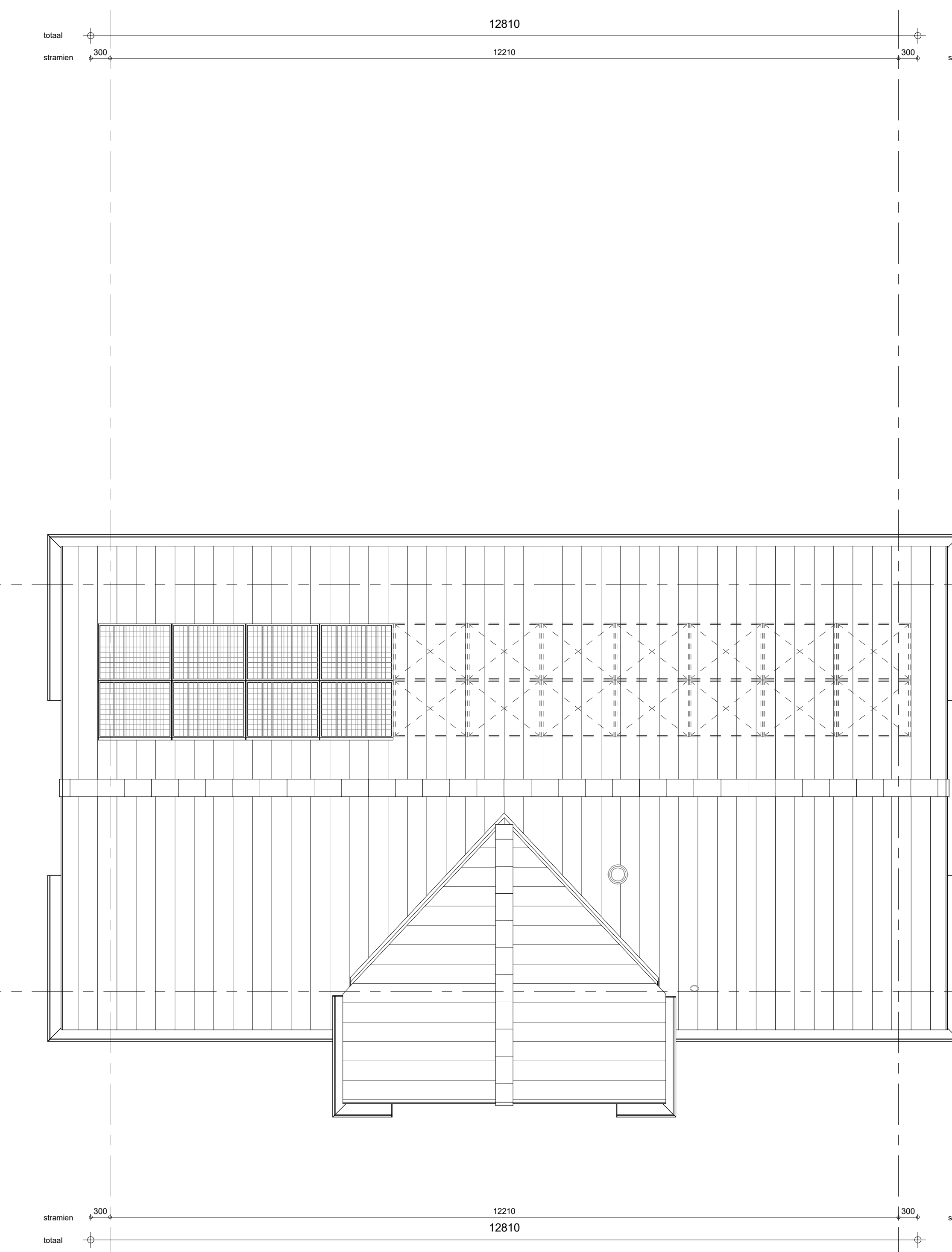
Dakaanzicht 1 : 50
