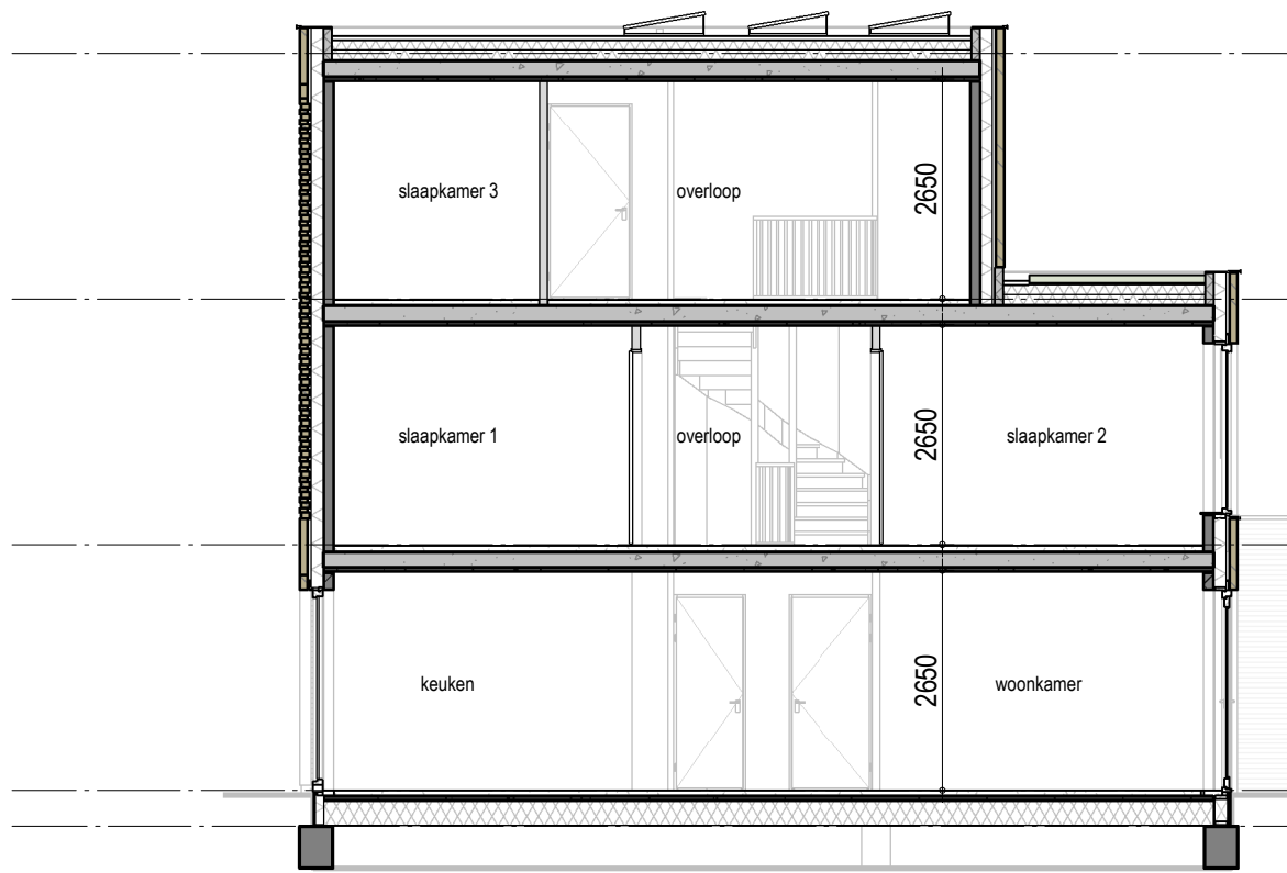
Doorsnede 42B-42B
