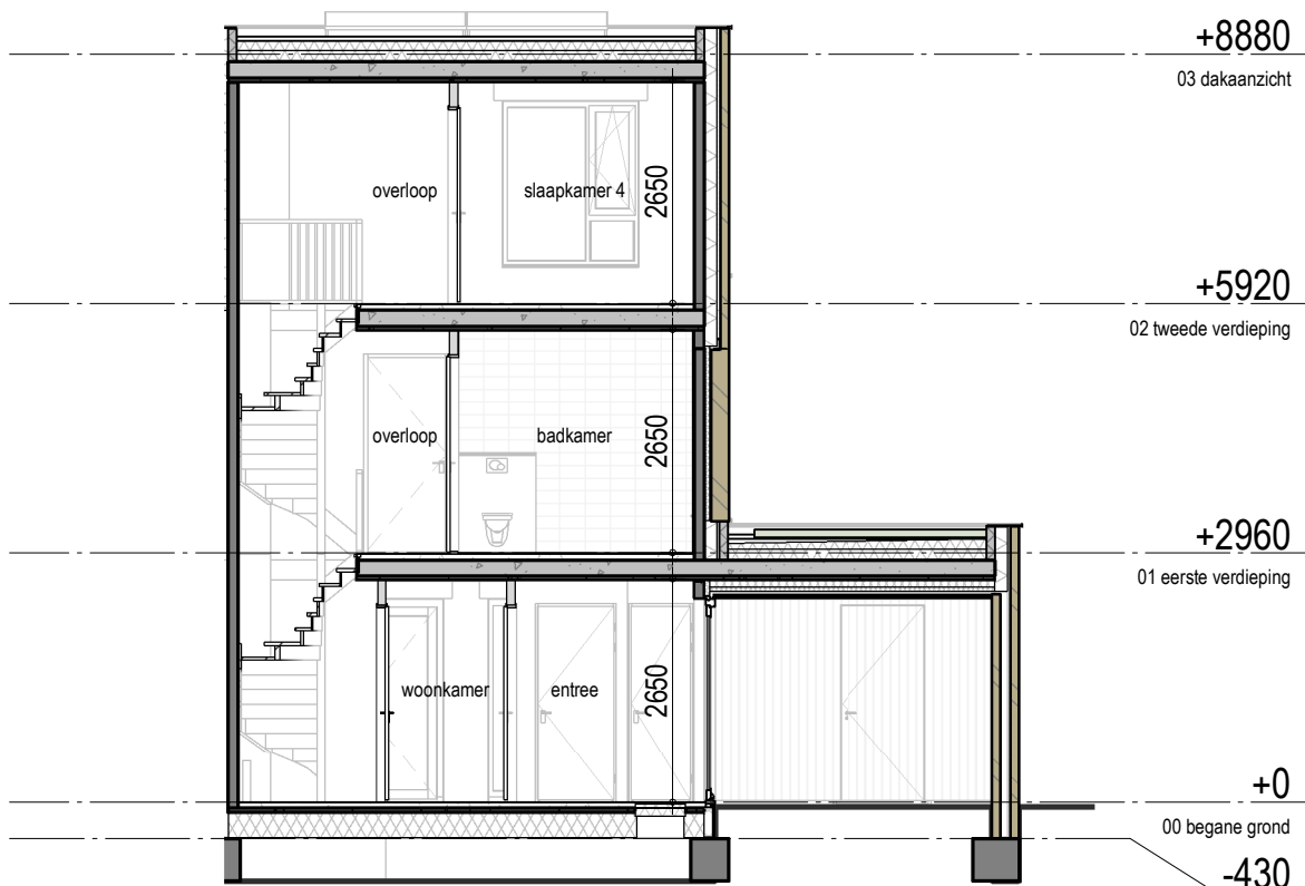
Doorsnede 42A-42A
