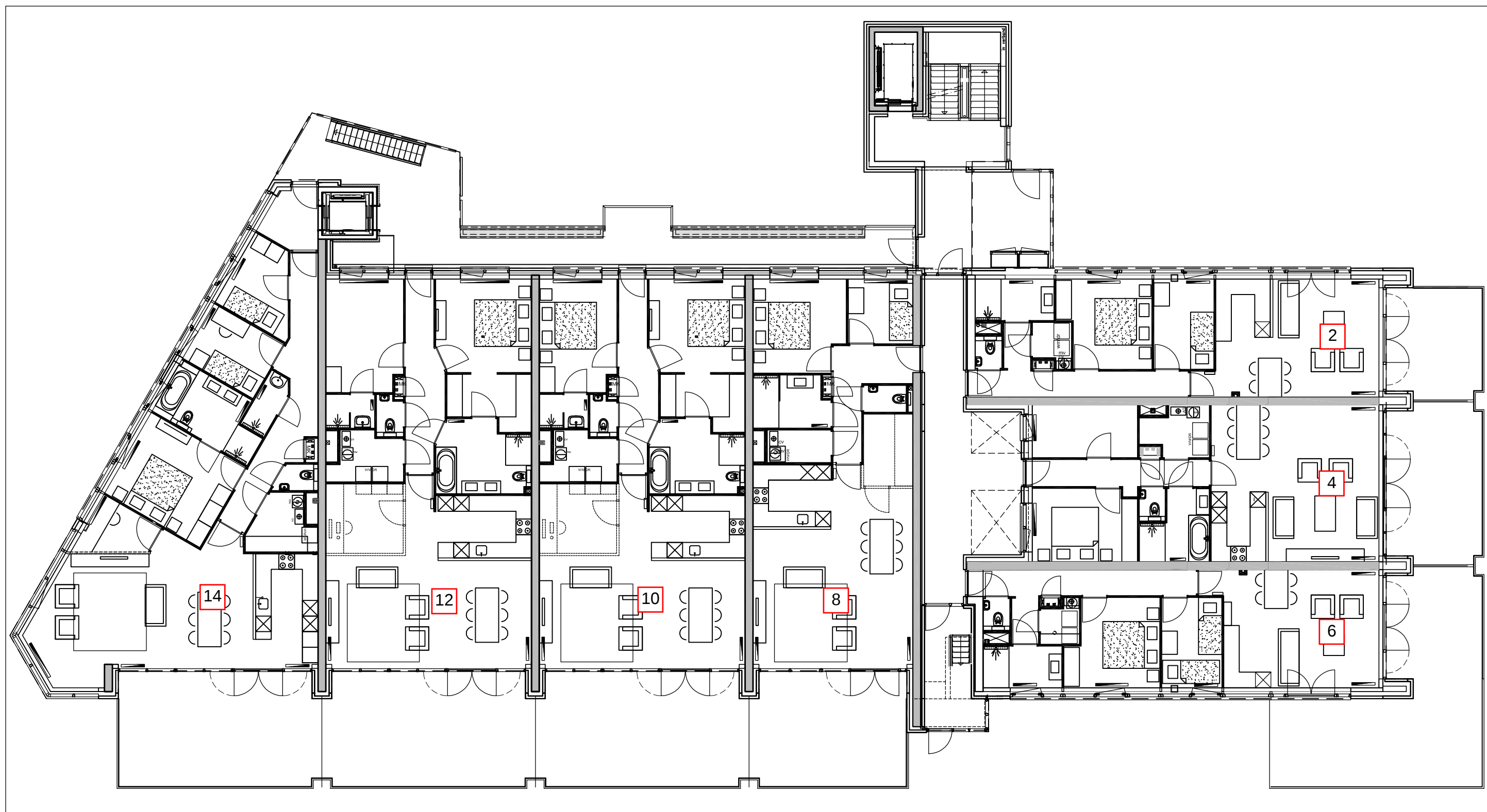
Begane grond
