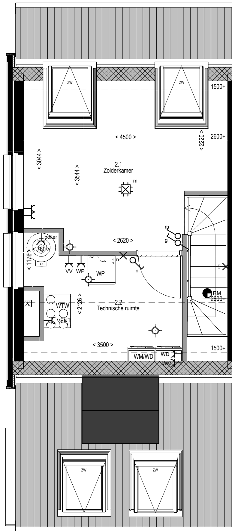
Tweede verdieping - BNR 01
