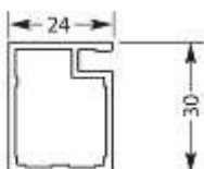
Kaderprofiel nr. 1005
