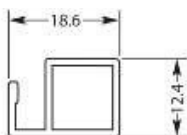
Kaderprofiel nr. 1010/F0
