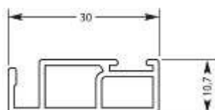
H2-A: Kaderprofiel nr. 1020
