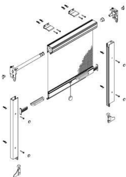
Montage ODD
