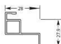
Kaderprofiel nr. 1050/28mm
