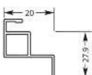
Kaderprofiel nr. 1065/20mm
