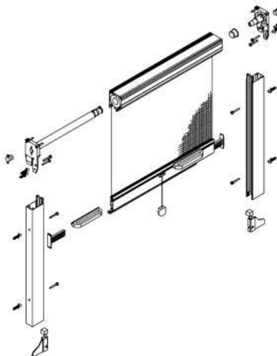
Montage IDD
