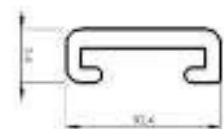
H1-D: Borstelprofiel nr. 1099
