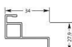
Kaderprofiel nr. 1055/34mm
