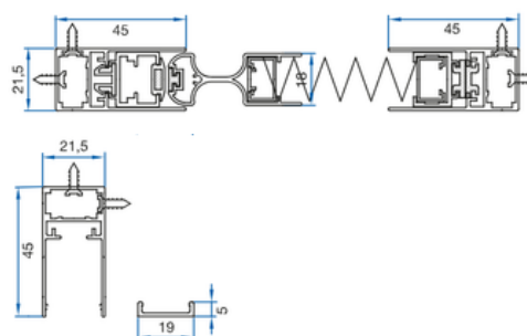
Opbouw
