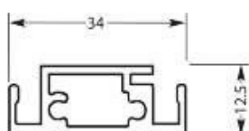
Tussenprofil nr. 1090 Sprosseprofil Nr. 1090 Midbar profile No. 1090
