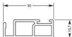
H1-A: Kaderprofil nr. 1020 Rahmenprofil Nr. 1020 Frame profile No. 1020
