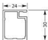
Kaderprofiel nr. 1005 Rahmenprofil Nr. 1005 Frame profile No. 1005
