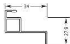
Kaderprofiel nr. 1055/34mm Rahmenprofil Nr. 1055/34mm Frame profile No. 1055/34mm
