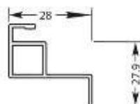
Kaderprofiel nr. 1050/28mm Rahmenprofil Nr. 1050/28mm Frame profile No. 1050/28mm
