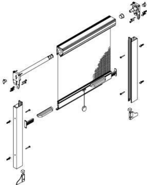
Montage IDD Montage in der Laibung Recess fixing
