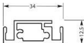
Tussenprofiel nr. 1090 Sprosseprofil Nr. 1090 Midbar profile No. 1090
