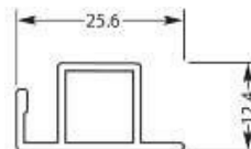
Kaderprofiel nr. 1003/F7 Rahmenprofil Nr. 1003/F7 Frame profile No. 1003/F7
