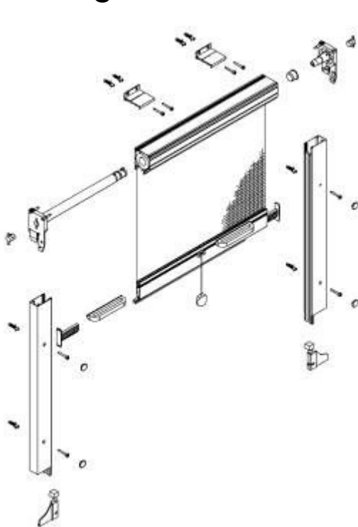
Montage ODD Montage auf der Laibung Frontal fixing
