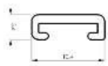
D1-C: Borstelprofiel nr. 1099 D1-C: Bürstprofil Nr. 1099 D1-C: Brush profile No. 1099
