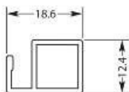
Kaderprofiel nr. 1010/F0 Rahmenprofil Nr. 1010/F0 Frame profile No. 1010/F0
