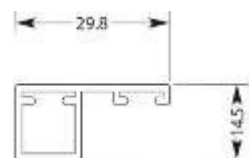
H2-B: Subframe nr. 1075 Montagerahmen Nr. 1075 Sub-frame No. 1075
