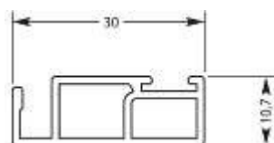
H2-A: Kaderprofiel nr. 1020 Rahmenprofil Nr. 1020 Frame profile No. 1020
