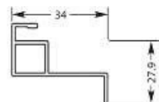
Kaderprofil nr. 1055/34mm Rahmenprofil Nr. 1055/34mm Frame profile No. 1055/34mm
