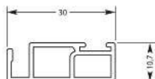
H1-A: Kaderprofiel nr. 1020 Rahmenprofil Nr. 1020 Frame profile No. 1020
