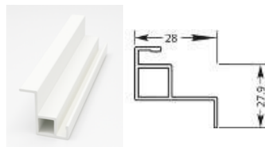
Kaderprofiel nr. 1050/28mm Rahmenprofil Nr. 1050/28mm Frame profile No. 1050/28mm
