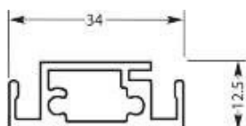
Tussenprofil nr. 1090 Sprosseprofil Nr. 1090 Midbar profile No. 1090
