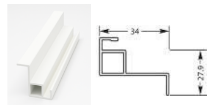
Kaderprofiel nr. 1055/34mm Rahmenprofil Nr. 1055/34mm Frame profile No. 1055/34mm
