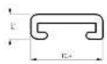
D1-C: Borstelprofil nr. 1099 D1-C: Bürstprofil Nr. 1099 D1-C: Brush profile No. 1099
