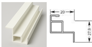
Kaderprofiel nr. 1065/20mm Rahmenprofil Nr. 1065/20mm Frame profile No. 1065/20mm
