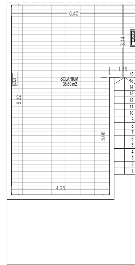
CUBIERTA
