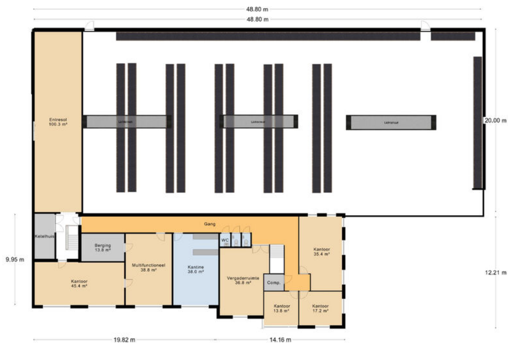
1e Verdieping
