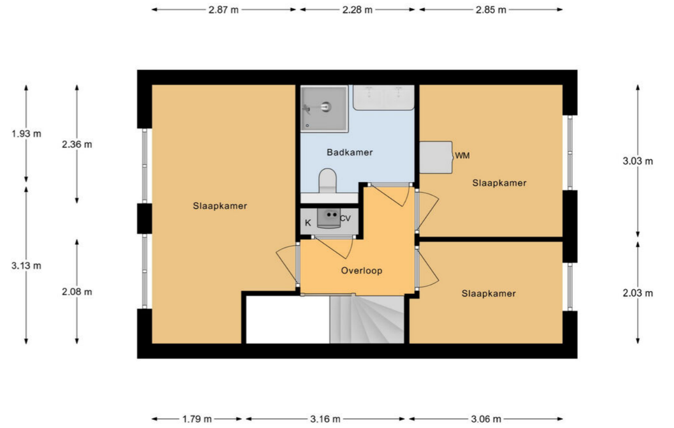
1e Verdieping
