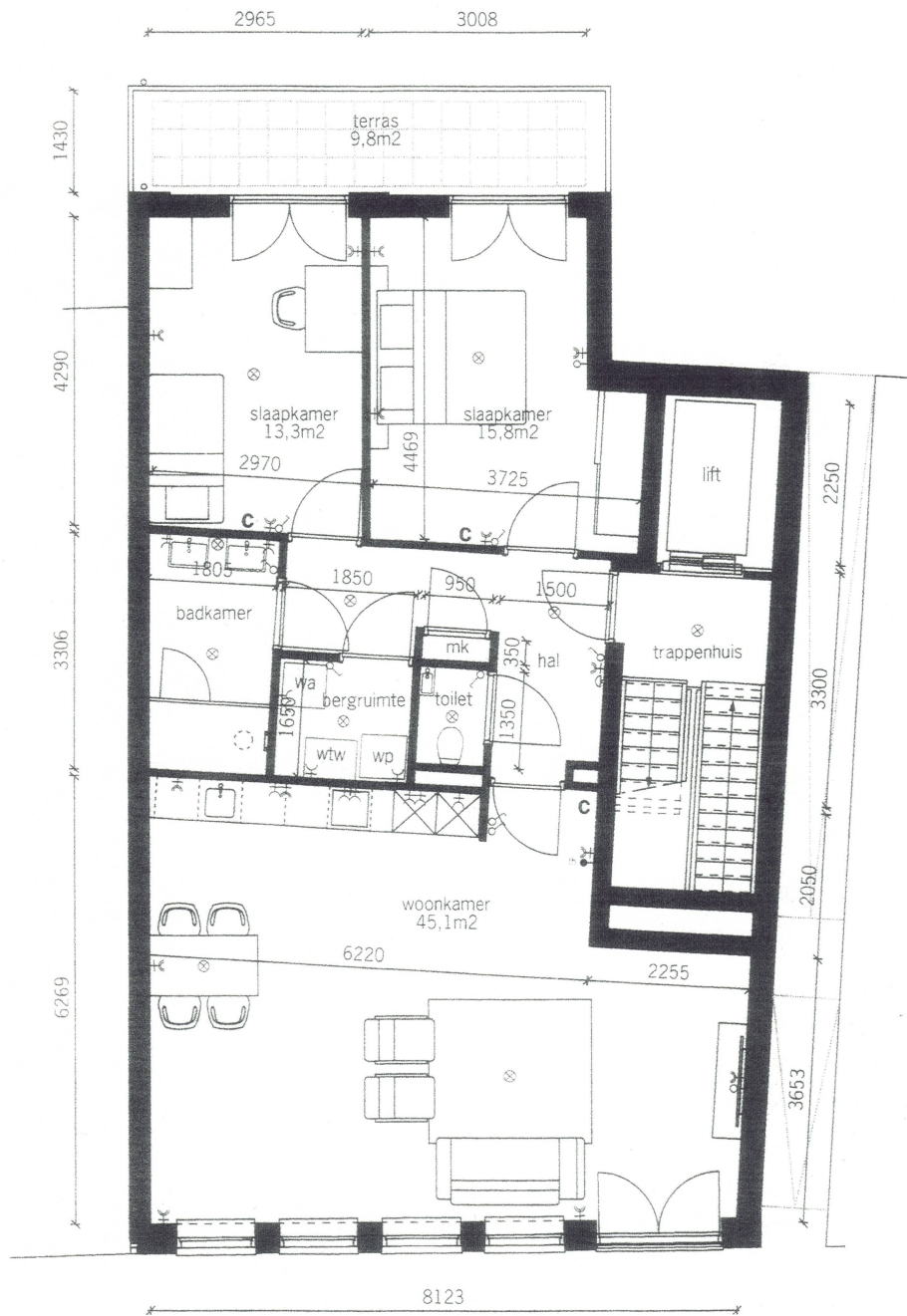
Appartementgebouw Sluisweg Dordrecht | Plattegrond 1e verdieping met woningnummer 01
