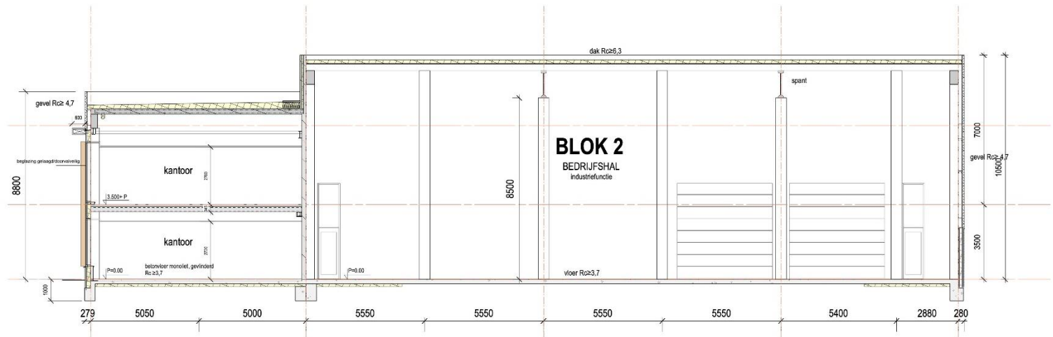
DOORSNEDE A-A
