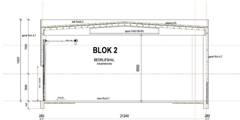
DOORSNEDE B-B
