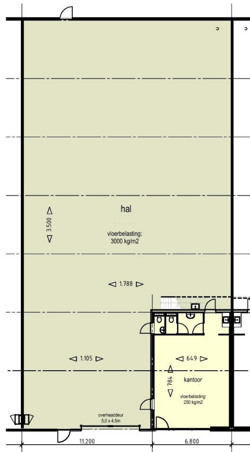
totaal plattegrond
