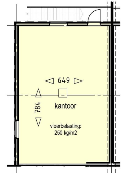
1e verdieping
