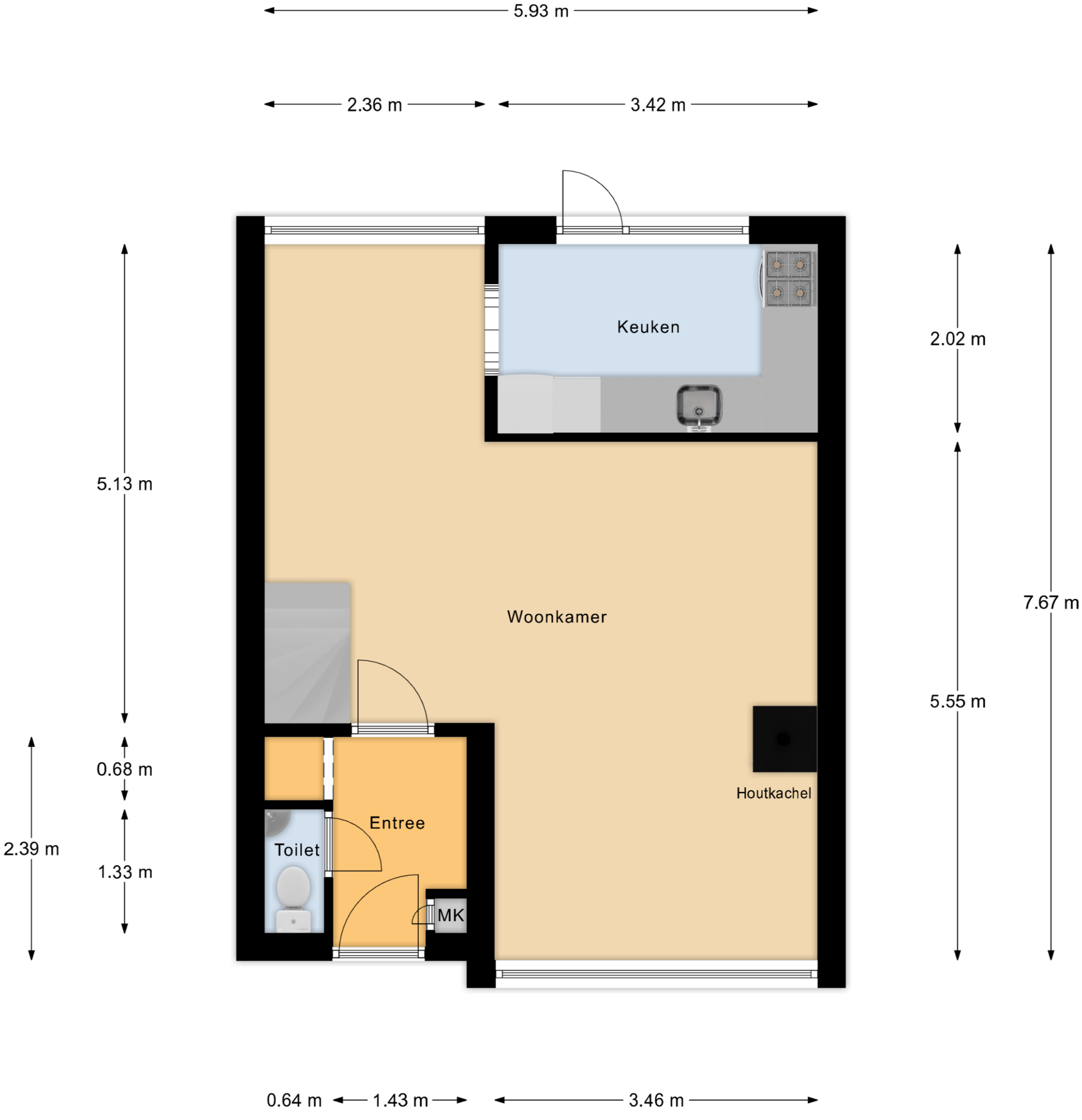
Begane Grond
